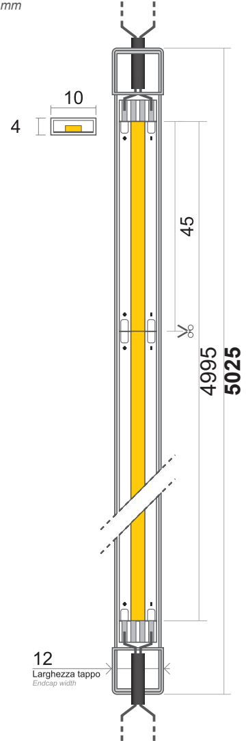
Uscita cavo / Cable output: IN/OUT Lunghezza cavi / Cables length: 200mm
